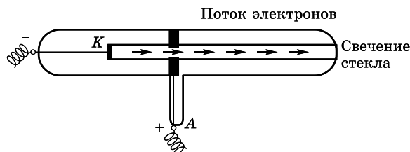
Рис. 1.1. Катодная трубка Томсона
