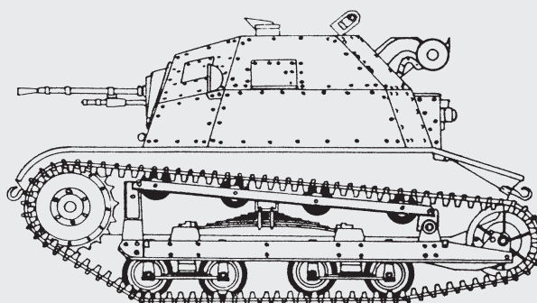
Танкетка ТКС
