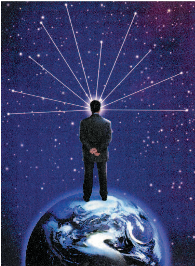
Звезды в бесконечной стационарной Вселенной.
