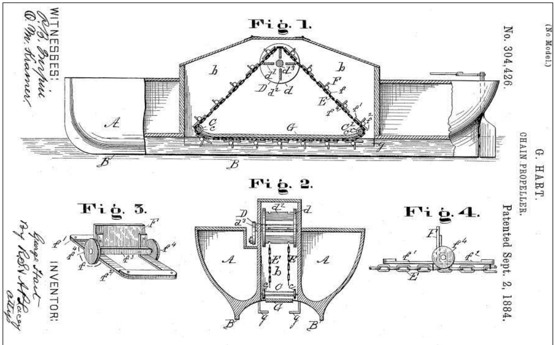
Патент Джорджа Харта от 1884 г. на «цепной движитель» для судна (США)
