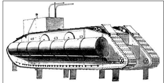
Британский опытный плавающий танк на основе тяжелого «десантного» танка Mk IX «ромбовидной» схемы. Обратим внимание на цистерны-поплавки по бортам и лопатки-гребки, шарнирно укрепленные на траках гусениц
