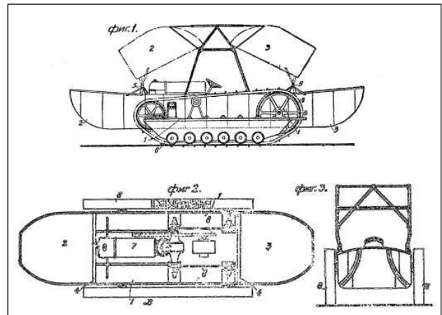
Рисунки «водосухопутной повозки» из патента Н.С. Ветчинкина от 1929 г. Гусеницы служили движителем на суше и на плаву, водоизмещающий корпус имел откидываемые на шарнирах вверх носовую и кормовую части
