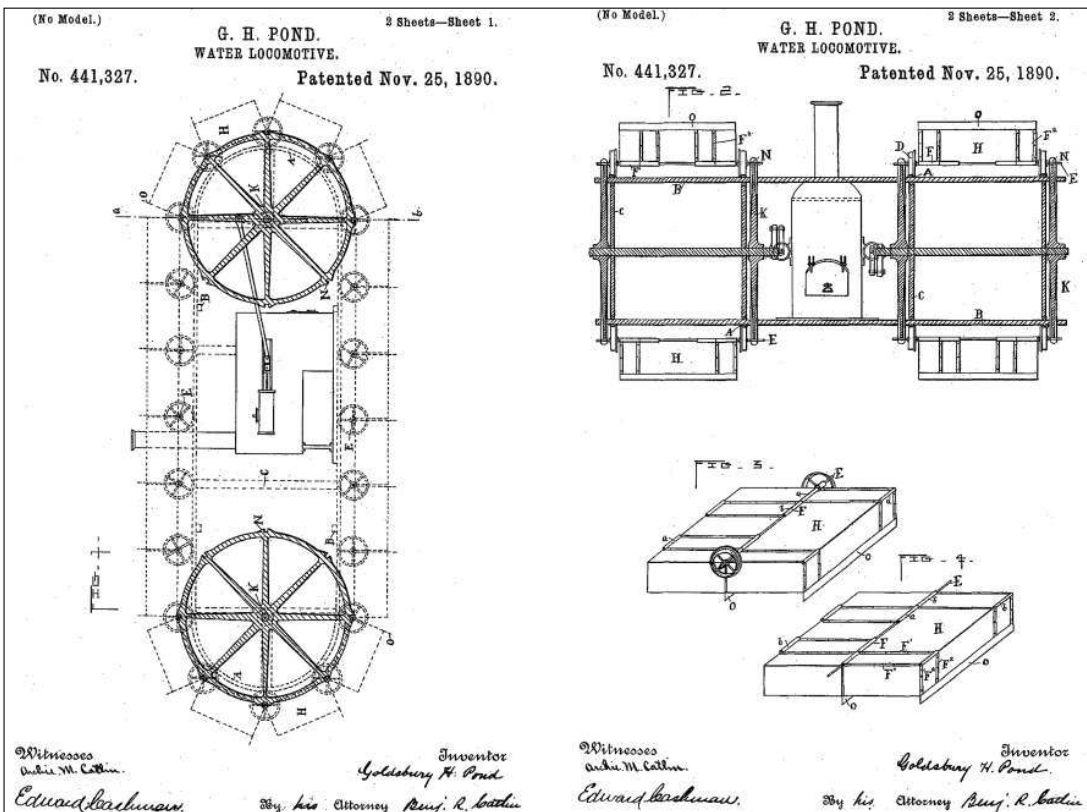
Патент Голдсбери Понда от 1890 г. на паровой «водный локомотив» с двумя гребными гусеницами, составленными из траков-понтонв (США)
