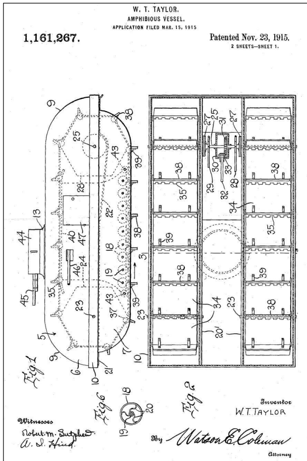
Патент на «амфибийное судно», полученный Уильямом Тейлором в 1915 г. (США). Движителем на суше и на плаву этой машине военного назначения должны были служить гусеницы
